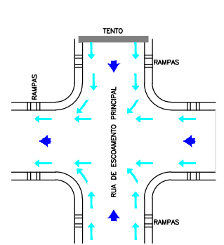
DETALHE ESCOAMENTO SUPERFICIAL NOS CRUZAMENTO
