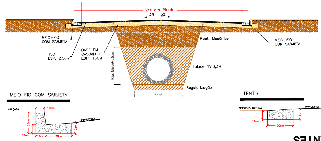
SEÇÃO TIPO DE PAVIMENTAÇÃO
