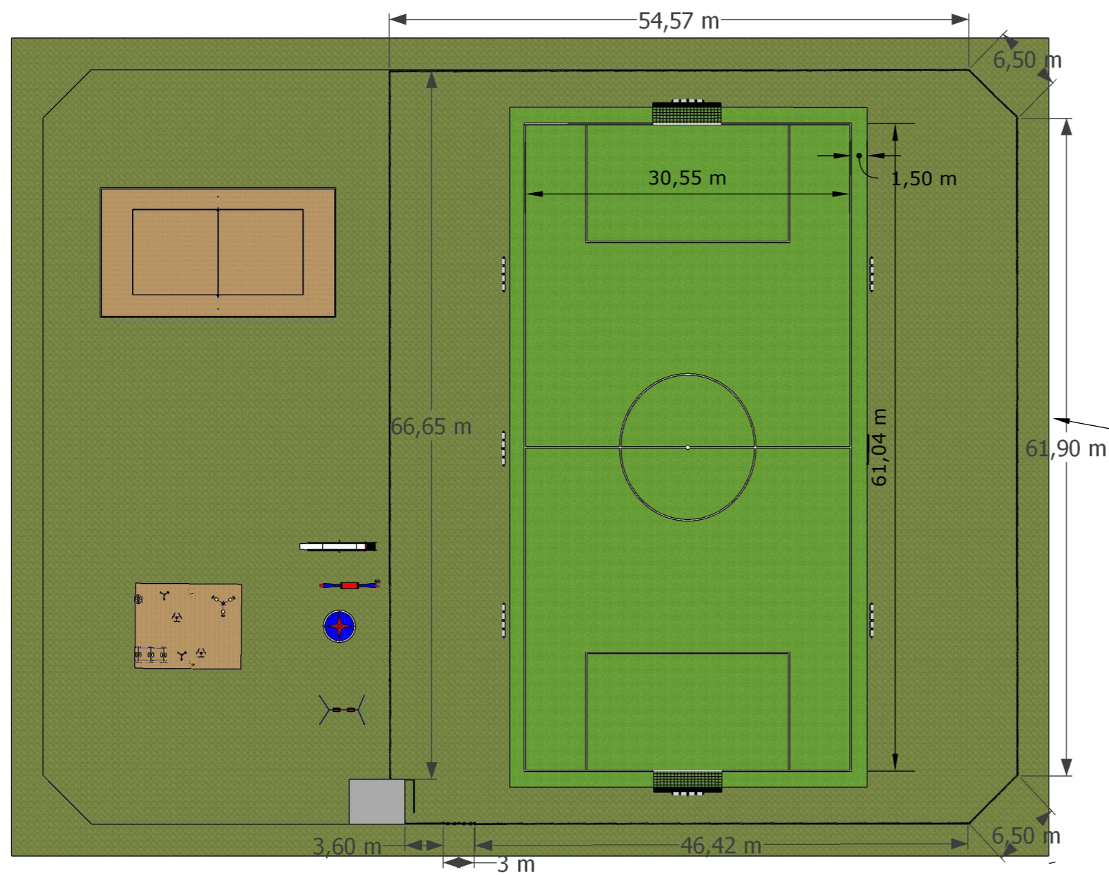
PLANTA BAIXA CAMPO DE FUTEBOL ESC:1/500
