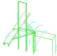
10 DETALHE 3D LIGACAO PERIS DE ACO P/ PILARES ESCALA 1/10
