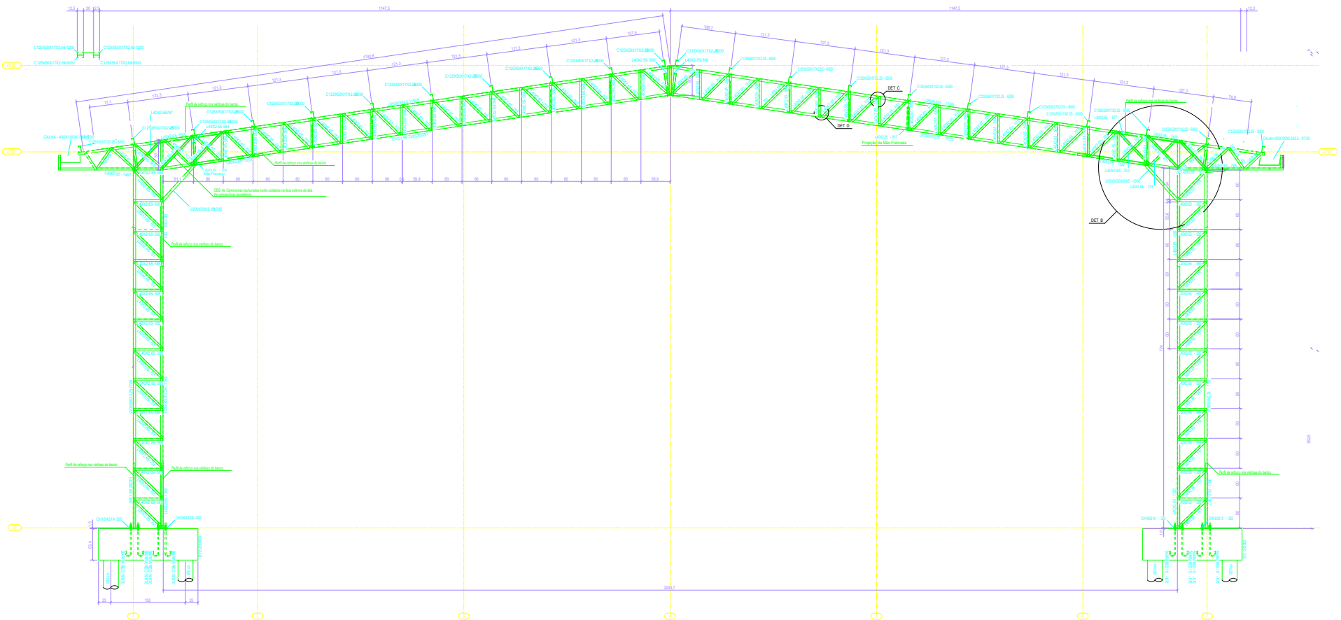
1 ELEVACAO DO EIXO B = EIXO C = EIXO D = EIXO E ESCALA 1/10
